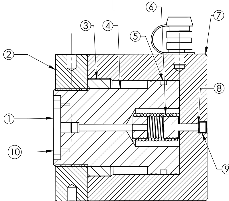
SECTION A-A SCALE 1 : 3
